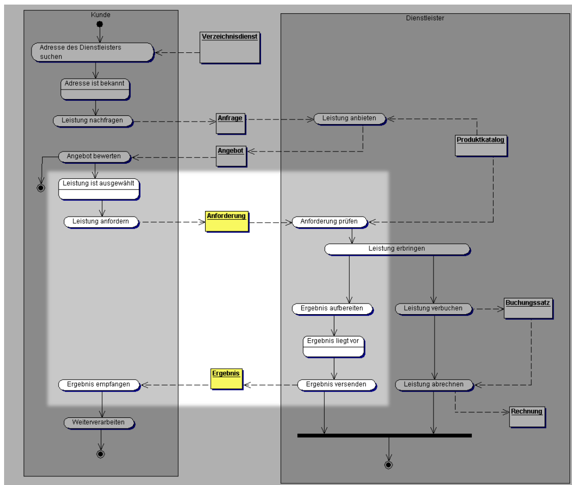
Bild 1-3 Das Referenzprozessmodell
