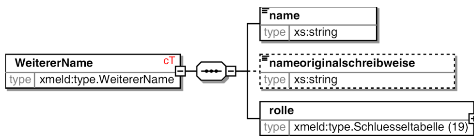
Bild 2-24 type.WeitererName
