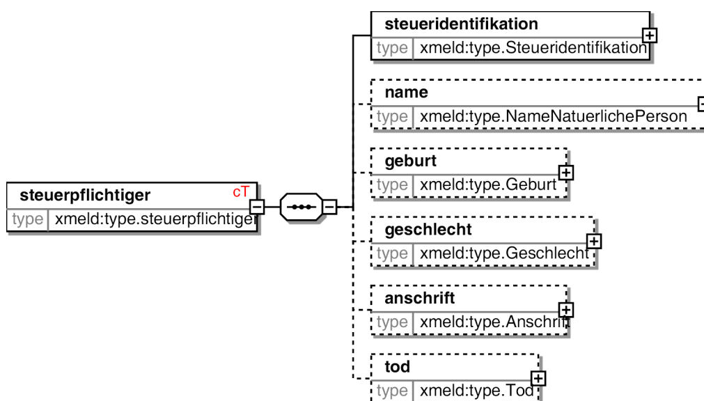
Bild 8-15 type.steuerpflichtiger
