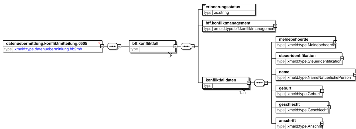
Bild 8-20 dateneuebermittlung.konfliktmitteilung.0505
