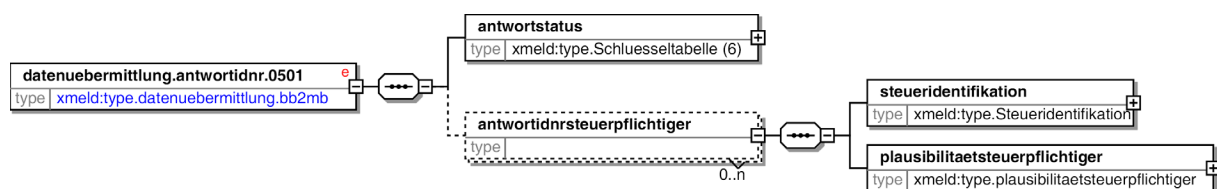
Bild 8-17 datenuebermittlung.antwortidnr.0501
