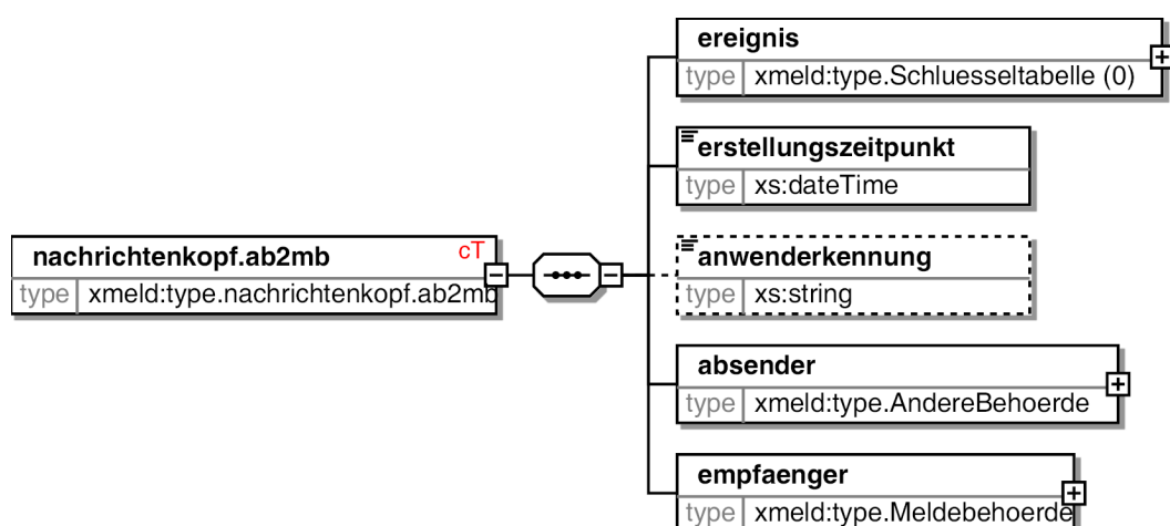
Bild 3-4 type.nachrichtenkopf.ab2mb
