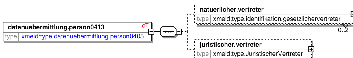
Bild 7-12 type.datenuebermittlung.person0413
