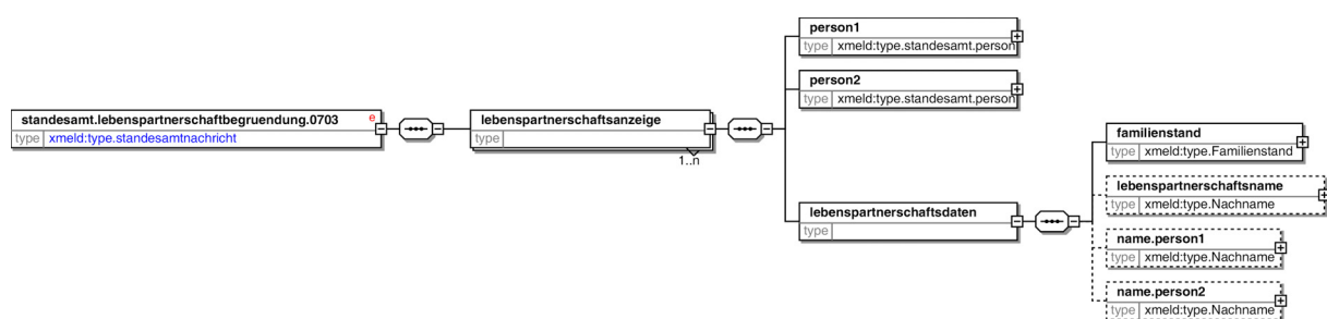
Bild 11-12 standesamt.lebenspartnerschaftbegrueudung.0703
