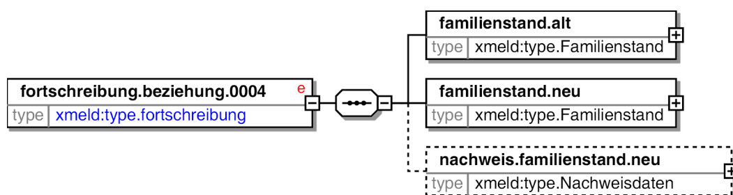
Bild 6-12 fortschreibung.beziehung.0004
