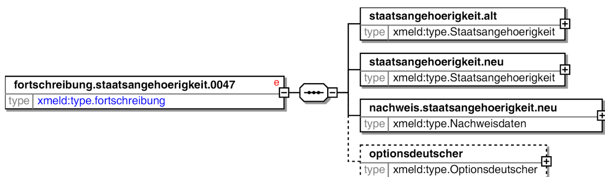
Bild 6-47 fortschreibung.staatsangehoerigkeit.0047
